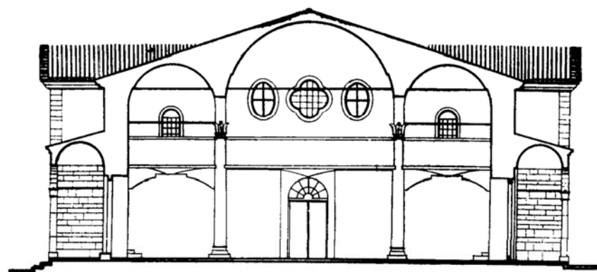
А. Напречен разрез
